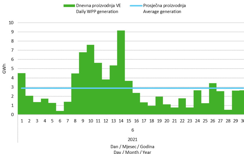
Slika 5 Dnevna proizvodnja svih vjetroelektrana u lipnju 2021. godine
