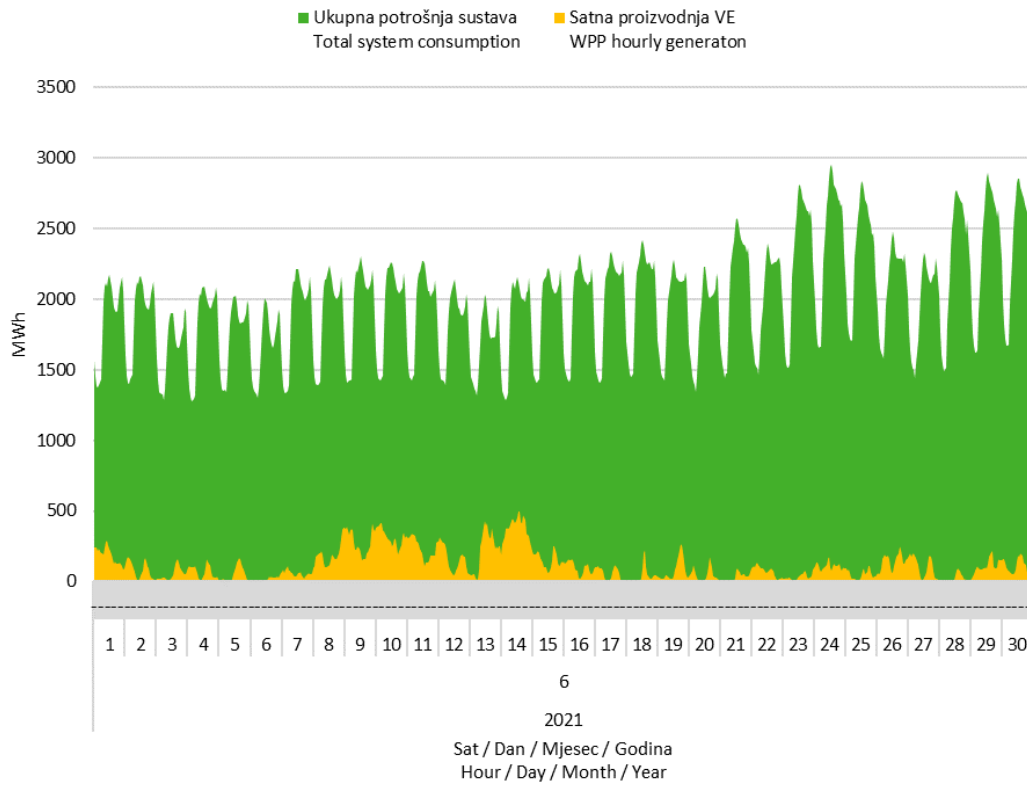
Slika 7 Usporedba satnog dijagrama opterećenja sustava i proizvodnje vjetroelektrana u lipnju 2021. godine
