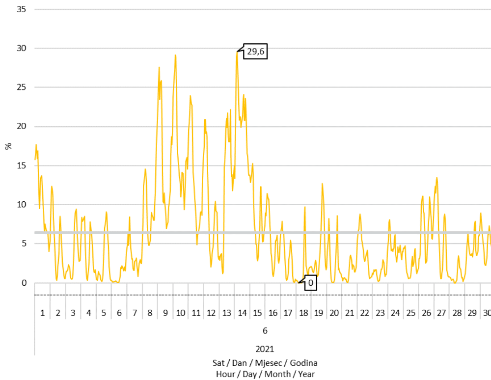
Slika 8 Udio proizvodnje vjetroelektrana u pokrivanju satnog opterećenja elektroenergetskog sustava u lipnju 2021. godine
