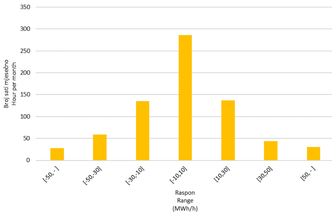
Slika 10 Statistička raspodjela satnih promjena proizvodnje VE u lipnju 2021. godine
