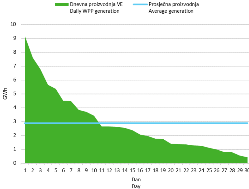
Slika 6 Krivulja trajanja dnevne proizvodnje vjetroelektrana u lipnju 2021. godine
