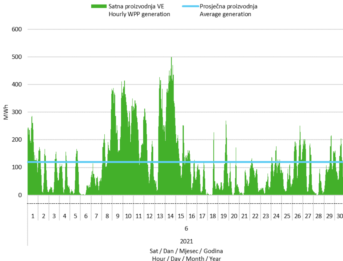
Slika 2 Satna proizvodnja svih vjetroelektrana u lipnju 2021. godine
