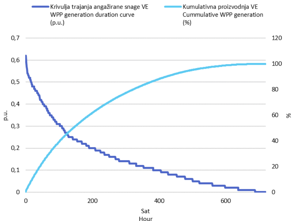
Slika 3 Krivulja trajanja angažirane snage svih VE i kumulativna proizvodnja VE u lipnju 2021. godine u jediničnim vrijednostima
