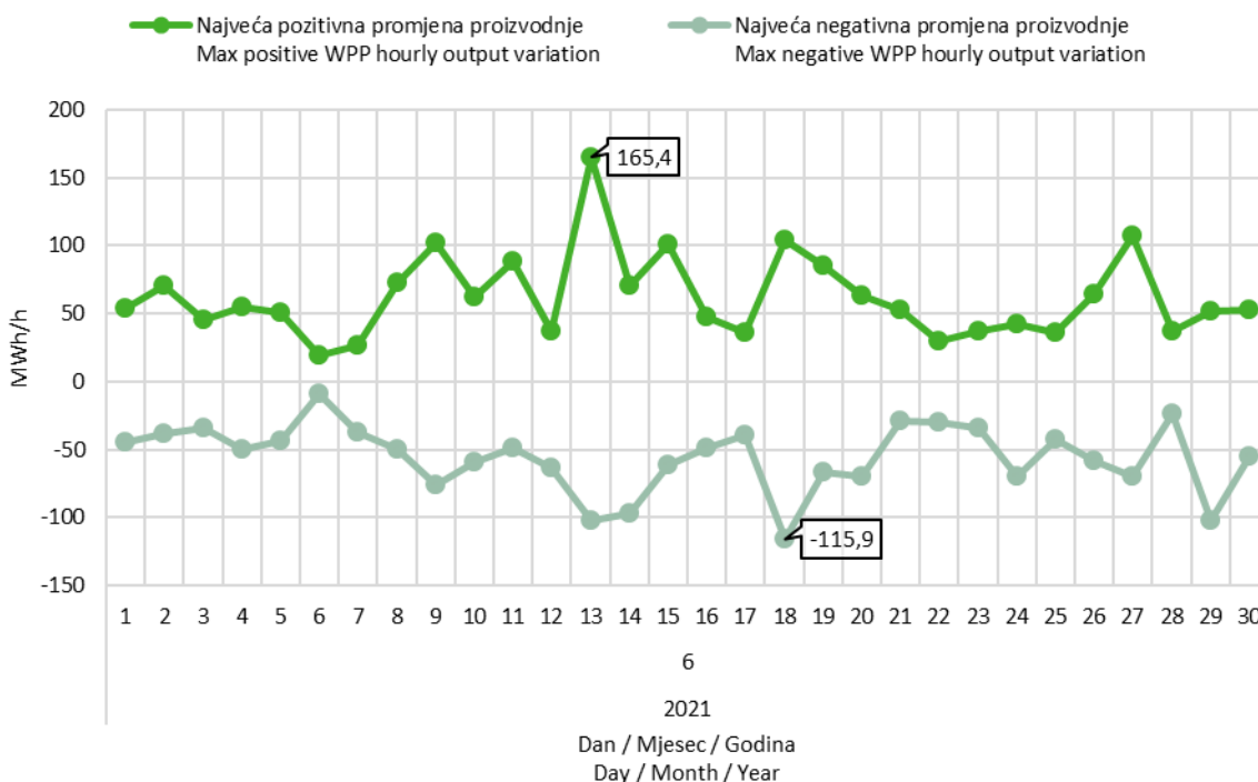
Slika 9 Maksimalna pozitivna i maksimalna negativna promjena satne proizvodnje VE u lipnju 2021. godine
